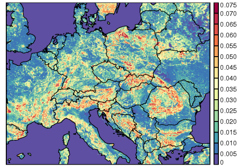
PCD : ALARO-pTKE+ISBA-2L+TEB S001RK_QCTEND 2011/03/03 z06:00 +6h
