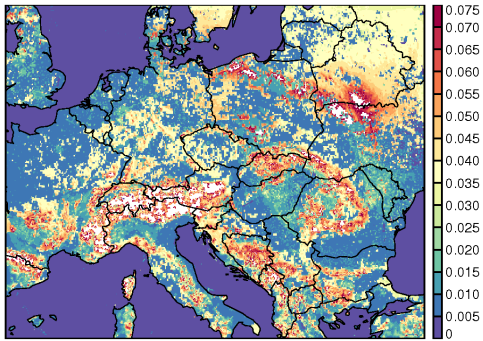
PCD : ALARO-pIKE S001RK_QCTEND 2011/03/03 z06:00 +6h
