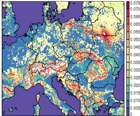
PCD : ALARO-TOUC S001RK_QCTEND 2011/03/03 z06:00 +6h
