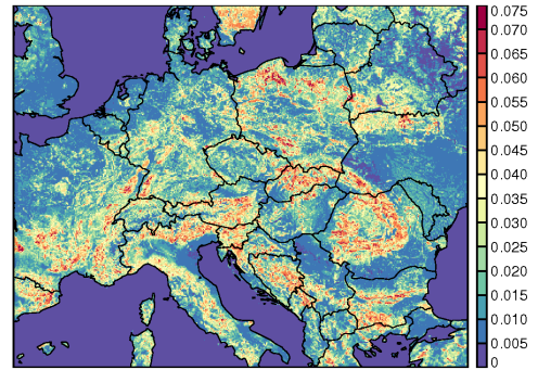
PCD : ALARO-pTKE+ISBA-2L S001RK_QCTEND 2011/03/03 z06:00 +6h
