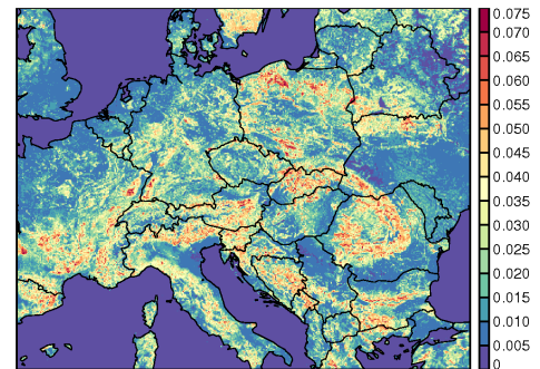
PCD : ALARO-pTKE+ISBA-2L+sfARP S001RK_QCTEND 2011/03/03 z06:00 +6h
